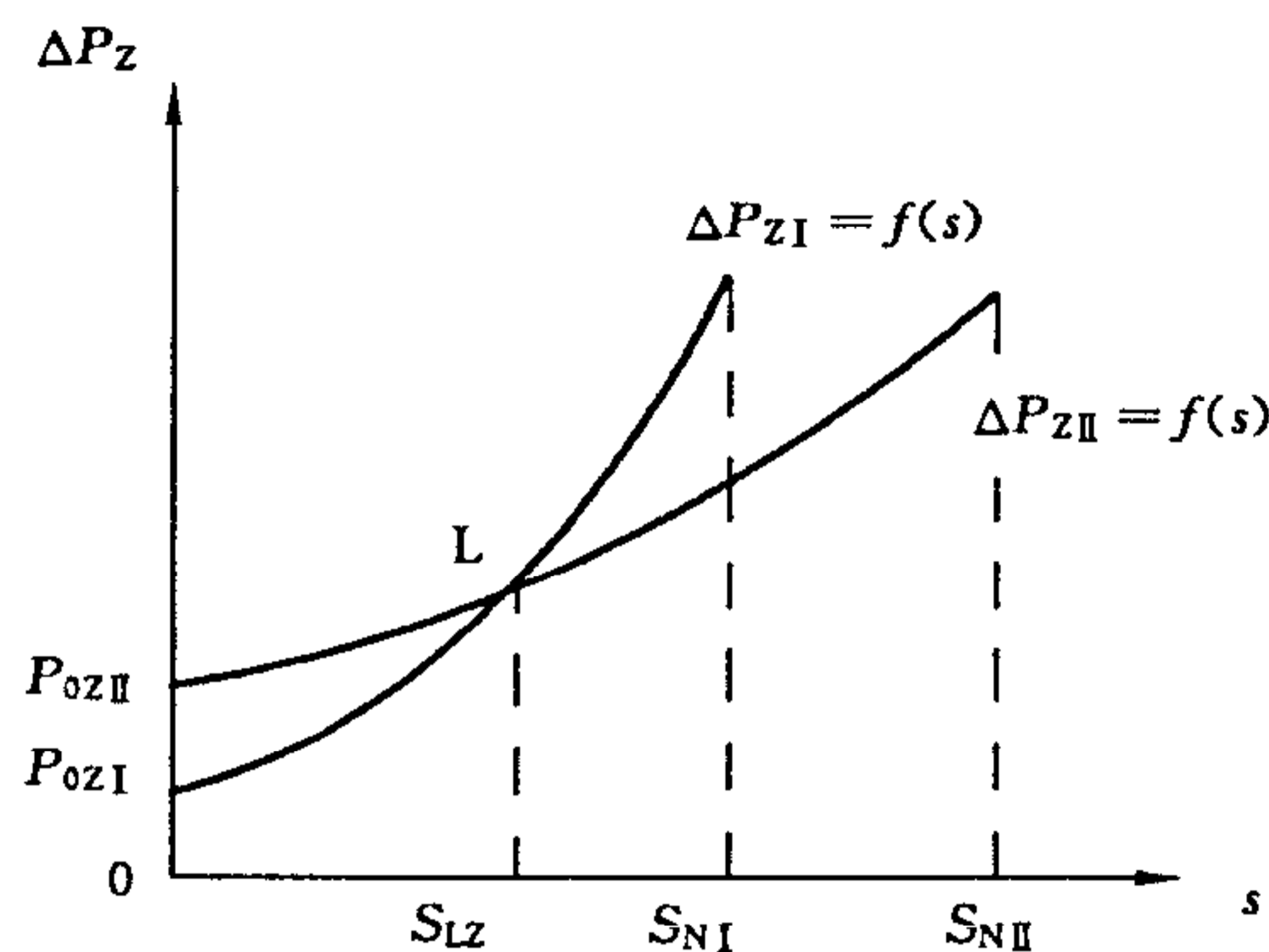
注: \Delta P_{zI} = f(s) 与 \Delta P_{zII} = f(s) 分别为变压器两种组合方式综合功率损耗 \Delta P_z 与负载视在功率 S 的函数特性曲线,两条曲线交点 L 的横坐标 S_{LZ} 即为两种组合运行方式的临界综合负载视在功率。
